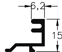
909 - Contravidrio peso: 0,16 Kg/m
